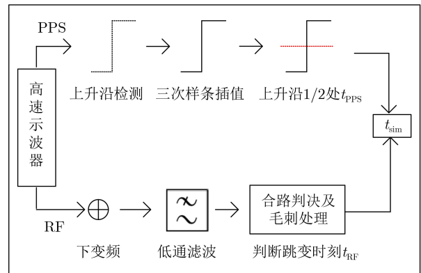
图3 采样数据相干解调处理算法原理
