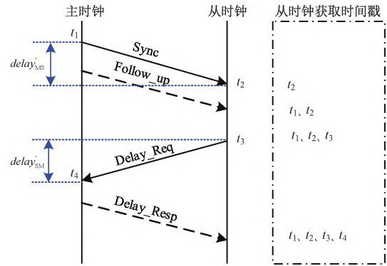
图3 PTP同步原理
