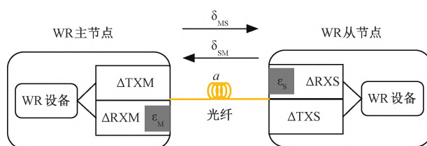
图1 WR链路同步模型
