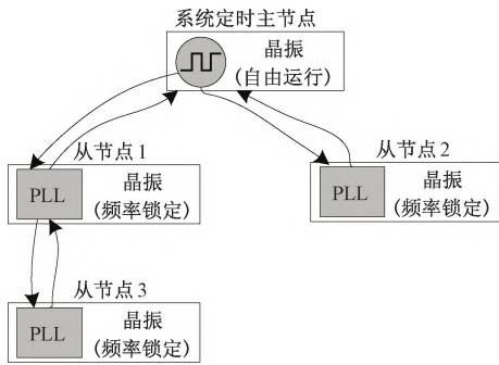
图2 频率同步原理
