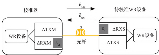
图4 基于校准器的整体校准模型
