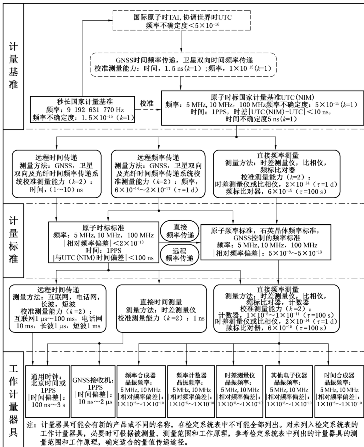
时间频率计量器具检定系统表框图
